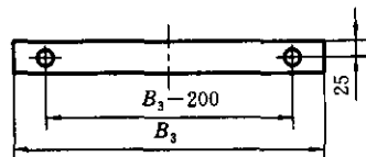
图 15 屏式仪表盘安装尺寸
