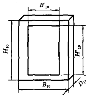
图 10 屏门基本尺寸示意图
