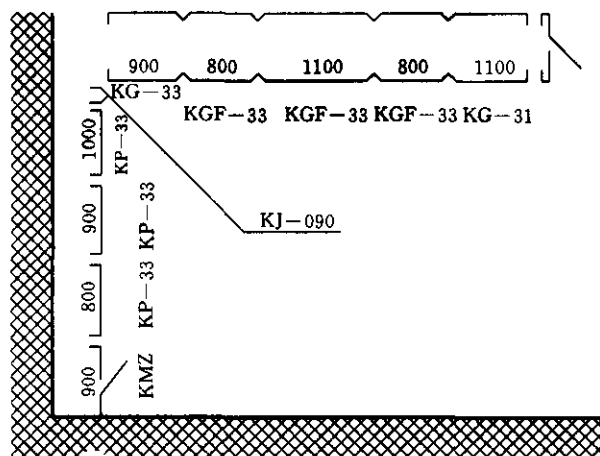
图 A1 组合使用图例
