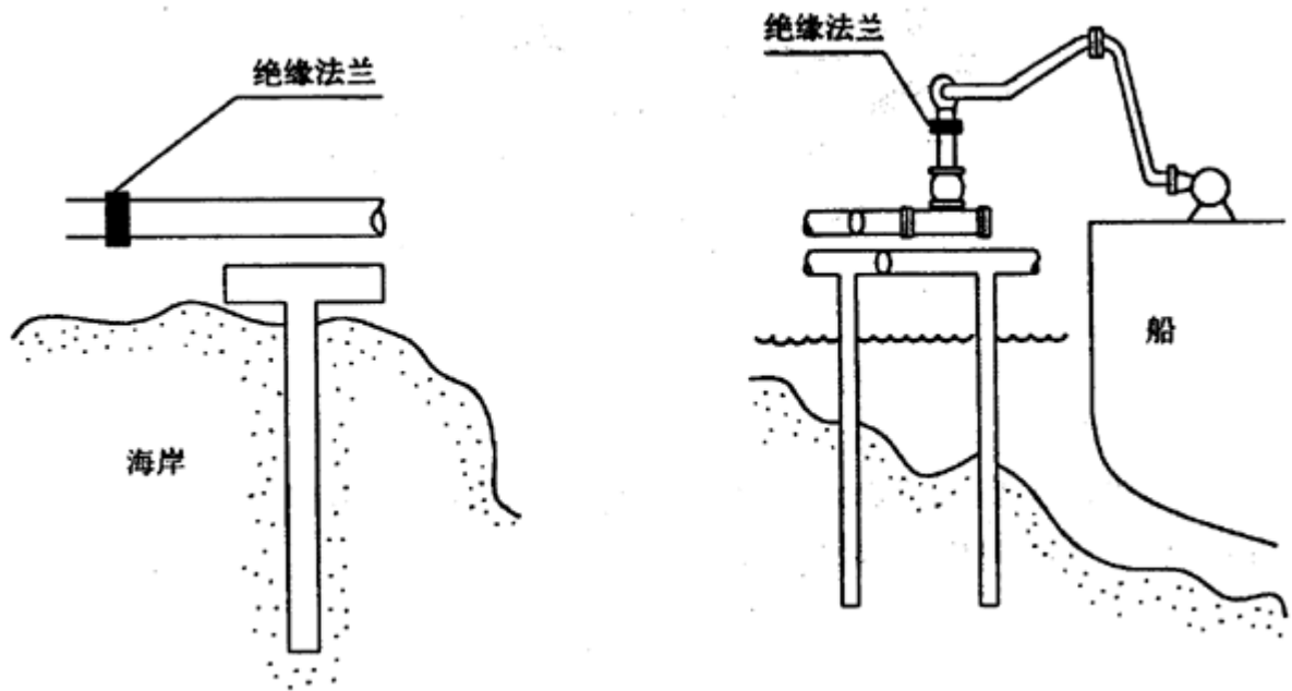
图 16 绝缘法兰使用示意
