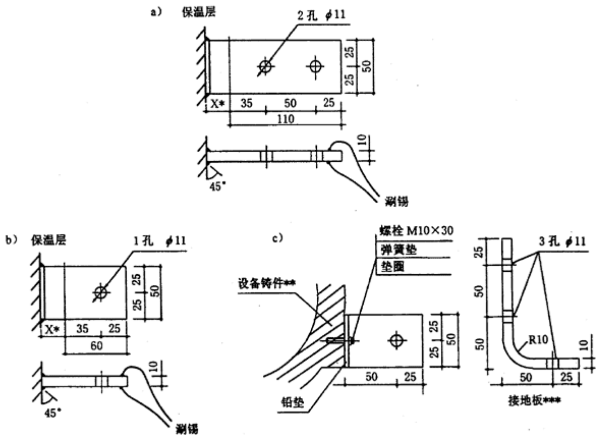
图 3 专用接地板组装示意图
