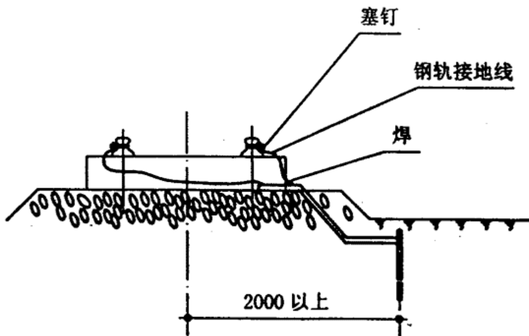
图 14 钢轨接地示意图。
