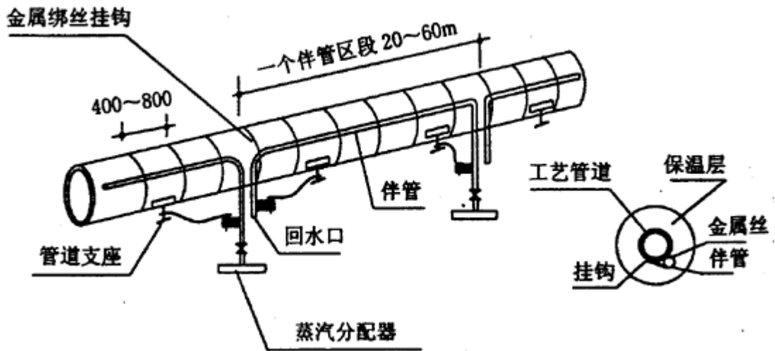
图10 蒸气伴管与工艺管道连接示意
