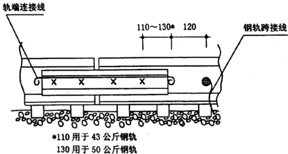
图 13 轨端跨接示意图
