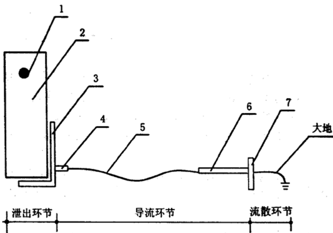
1——带电区 2——带电体的泄漏通道 3——设备支架、外壳 4——接地端子 5——接地支线 6——接地干线 7——接地体
