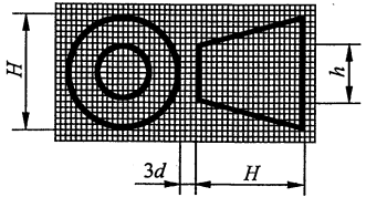
图 A.2 基本视图的配置(第三角画法)
