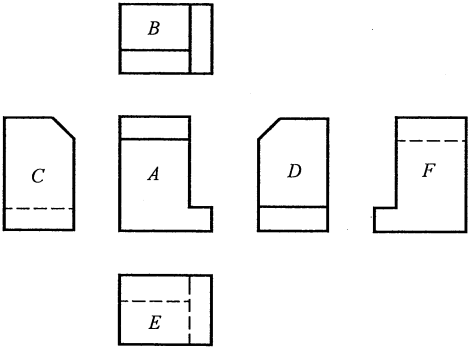
图 A.2 基本视图的配置(第三角画法)
