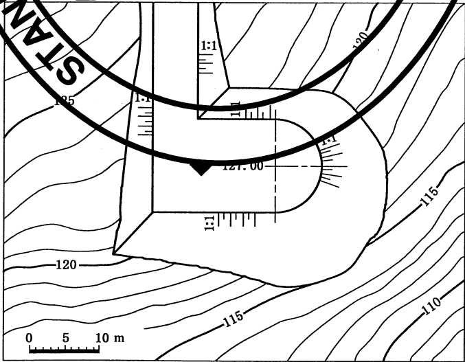
图 10 标高投影图
