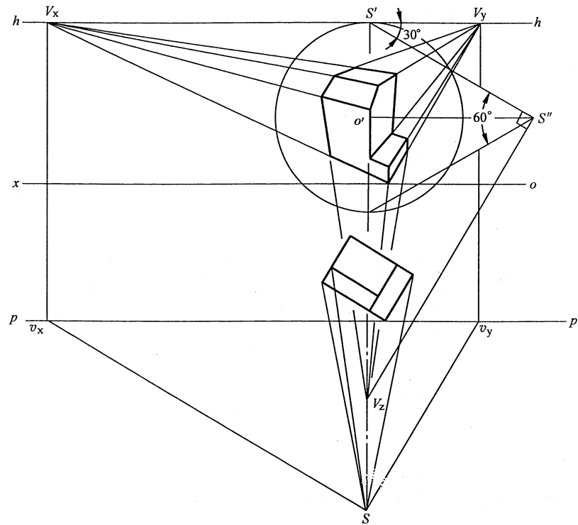
图 13 三点透视
