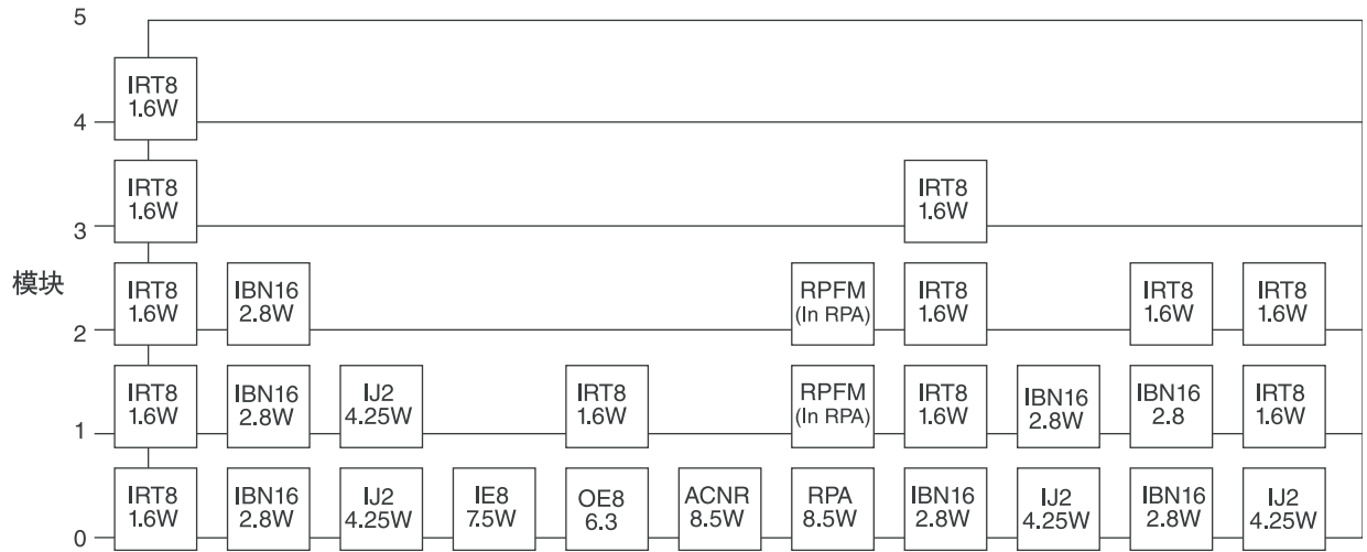
每个供电电源所供电的模块
