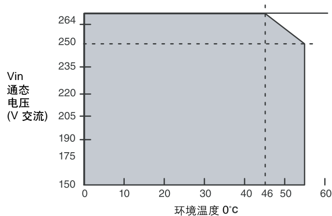
降额曲线
