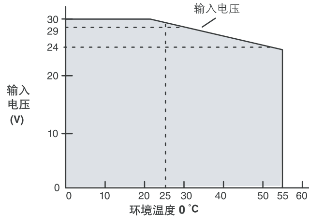
降额曲线
